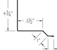
⑧ Universal Sidewall (SWcc)
