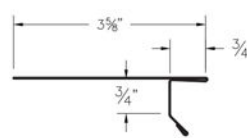
⑥① Drip Edge (DEcc)
