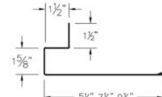
⑳ Door Trim (JTcc725 or JTcc925)
