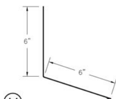
⑪ Universal Endwall (EWcc)
